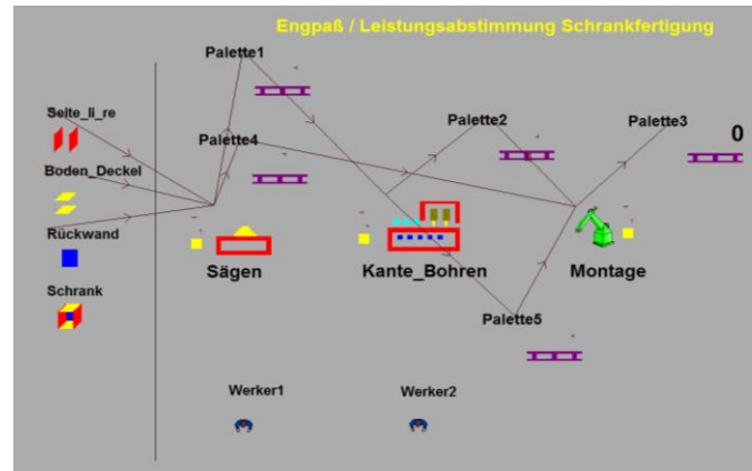
Fertigungsplanung mit witness®
